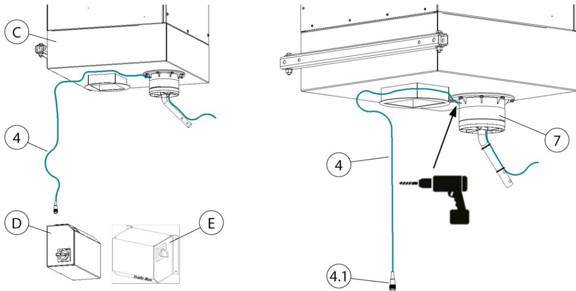
Abb. 17: Kabelverlegung – stationäres Gerät
