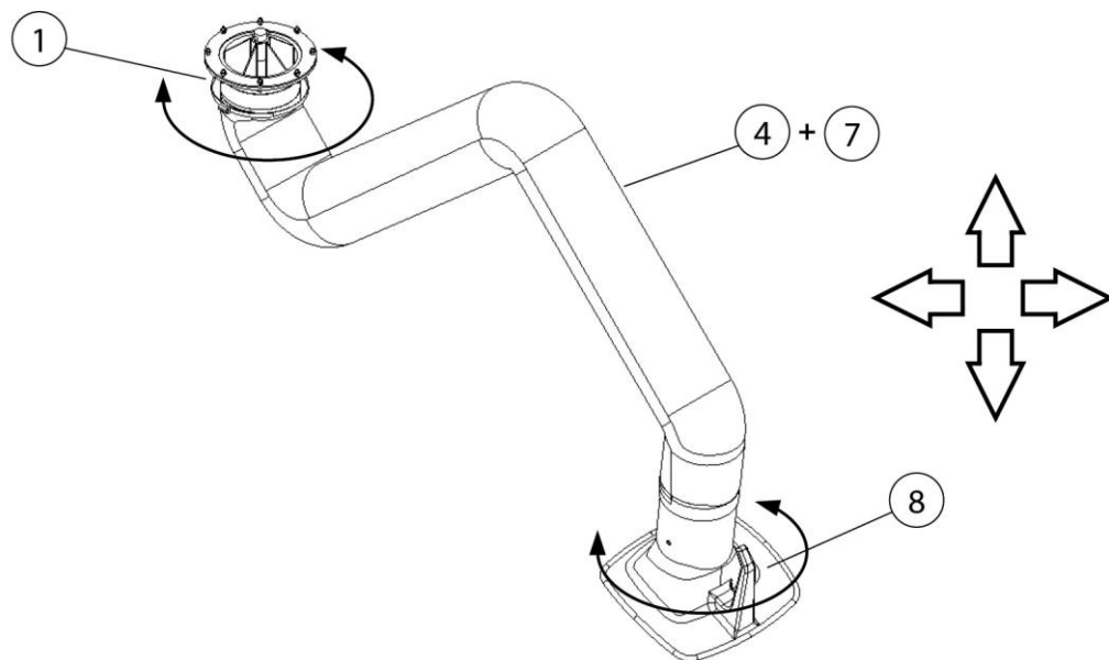
Abb. 1: Absaugarm – Funktionsbeschreibung
