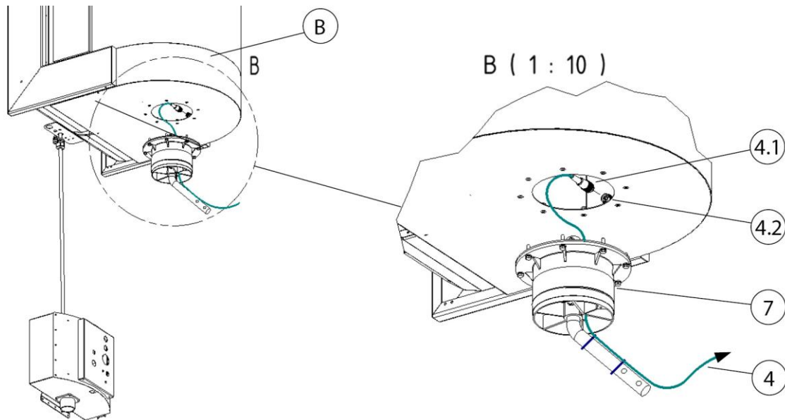
Abb. 16: Anschluss – stationäres Filtergerät
