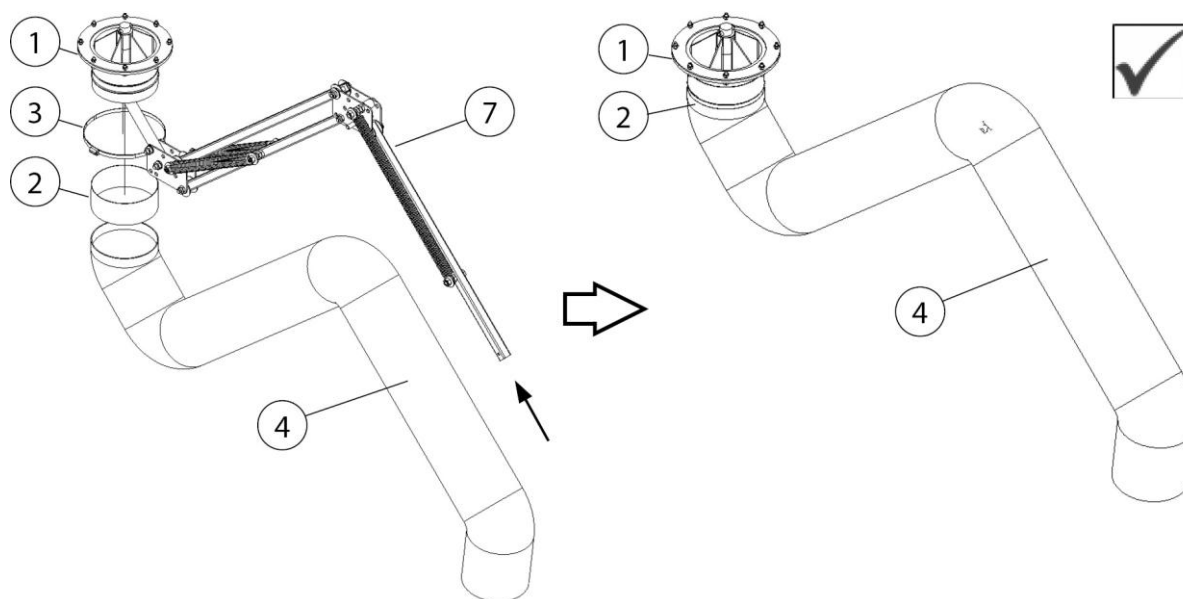
Abb. 13: Tragegestell/ Absaugarm
